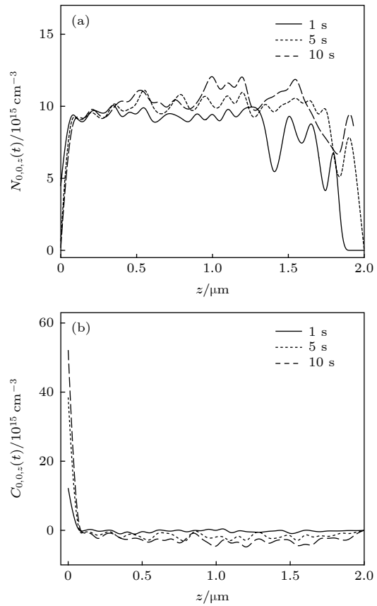
图 4 样品内部入射方向电荷分布 (a) 电子密度; (b) 净电荷密度
