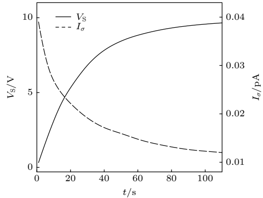
图 6 表面电位 V_S 和出射电子电流 I_\sigma 时变特性 Fig. 6. The surface potential V_S and emission current I_\sigma as function of time.
