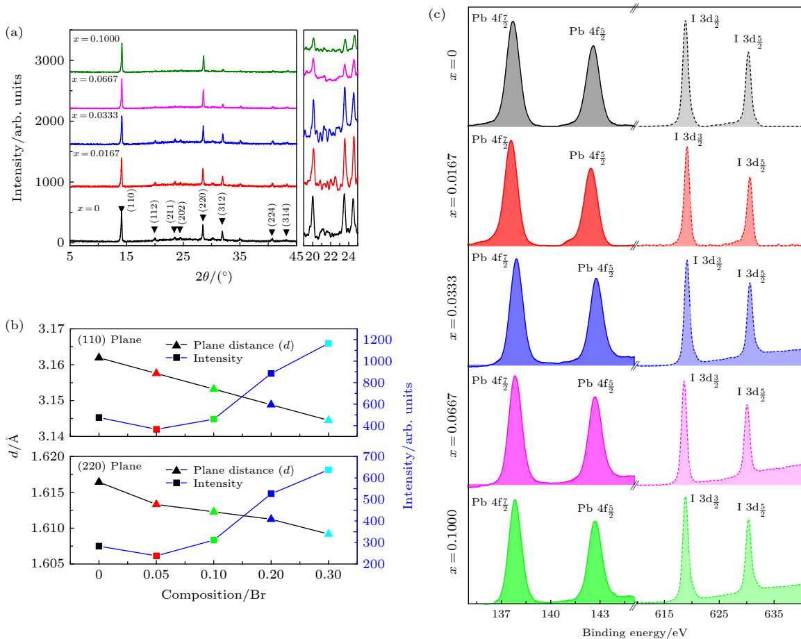
图 1 (a) 阴离子混合型钙钛矿 MAPb(Br x I 1-x ) 3 的 XRD 谱; (b) (110) 和 (220) 衍射峰强和晶面间距 d 随 Br 比例 x 的变化; (c) 不同 Br 比例的钙钛矿薄膜中 Pb 和 I 元素 XPS 谱
