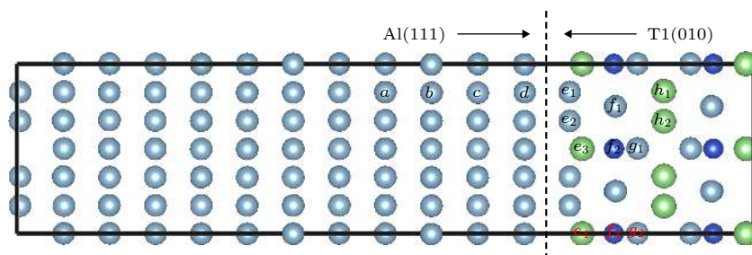
图 7 界面模型及其原子替换位置
