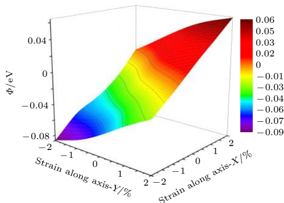
图 6 面 I 应变条件下电子功函数的变化
