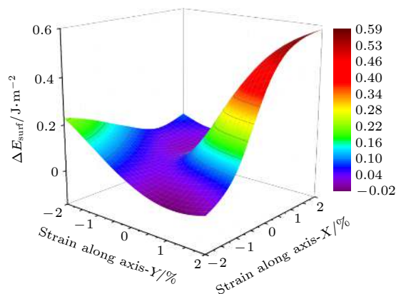
图 5 面 B 应变条件下表面能的变化
