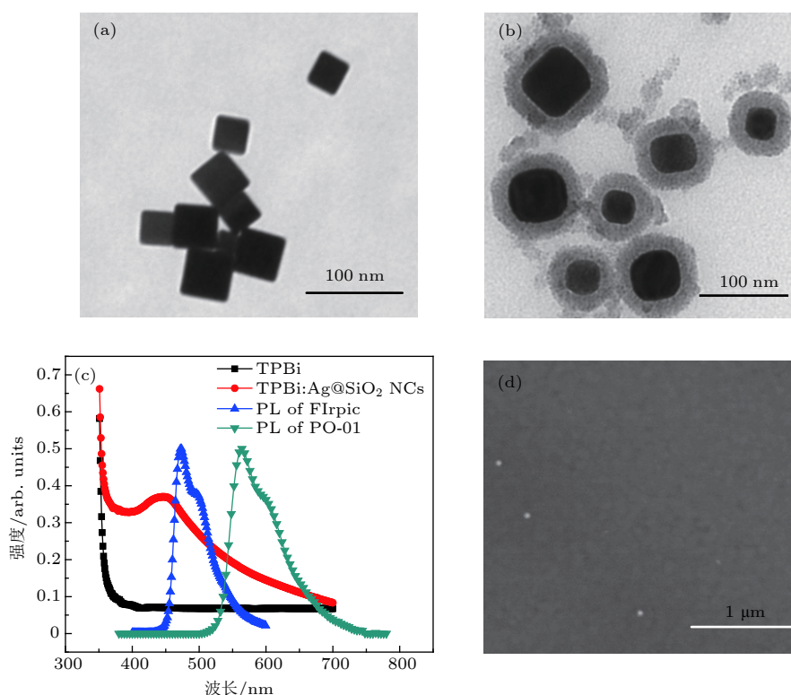
图 2 (a) 银纳米立方和 (b) Ag@SiO 2 NCs 的 TEM 图像; (c) TPBi 和掺有 Ag@SiO 2 NCs 的 TPBi 的吸收光谱, 以及 FIrpic 和 PO-01 的 PL 光谱; (d) 掺有 Ag@SiO 2 NCs 的 TPBi 表面的 SEM 图像
