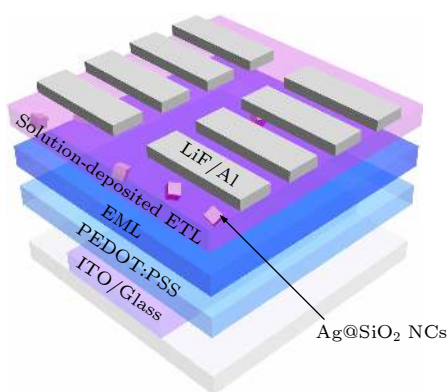
图 1 电子传输层中掺有 Ag@SiO 2 NCs 的 WOLED 器件结构示意图
