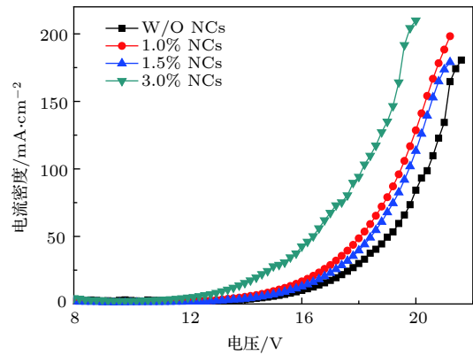
图5 单电子器件的电流密度-电压关系
