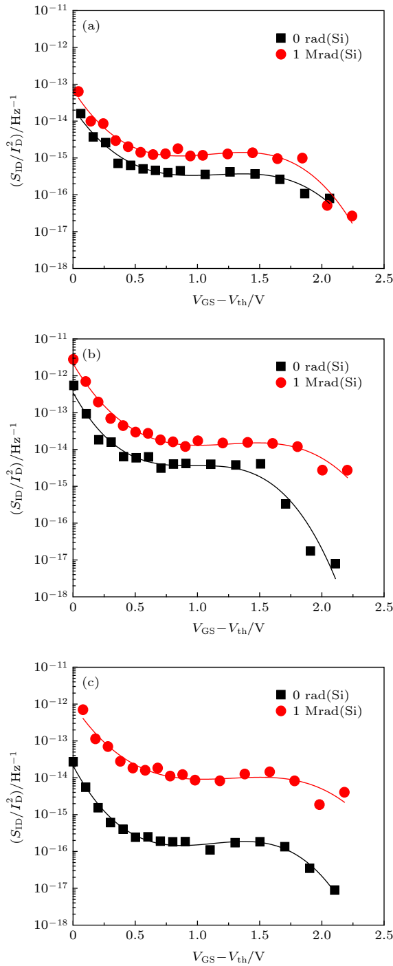
图6 AlGaIn/GaN HEMT 器件辐照前后沟道电流归一化噪声功率谱密度随过驱动电压的变化 (点: 测量值; 实线: 拟合值) (a) 关态; (b) 半开态; (c) 零偏
