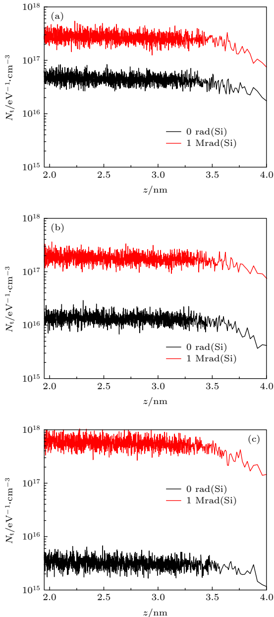
图 8 AlGaIn/GaN HEMT 器件辐照前后势垒层内陷阱电荷密度的空间分布 (a) 关态; (b) 半开态; (c) 零偏
