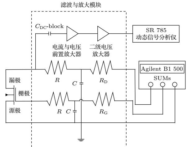
图 2 AlGaIn/GaN HEMT 器件的低频噪声测量系统 [17]
