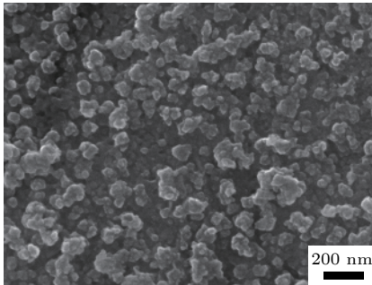
图 2 Tb 掺杂量为 x = 0.004 的高压烧结样品 (\text{Bi}_{1-x}\text{Tb}_x)_2(\text{Te}_{0.9}\text{Se}_{0.1})_3 的 FE-SEM 照片
