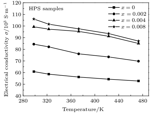
图 3 Tb 不同掺杂量的高压烧结样品的电导率随温度的变化
