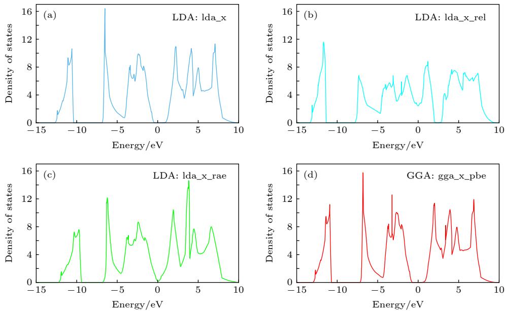
图 3 多种泛函计算的 GaAs 的态密度 (a) (b) (c) (d) Fig. 3. Calculated density of states (DOS): (a); (b); (c); (d).
