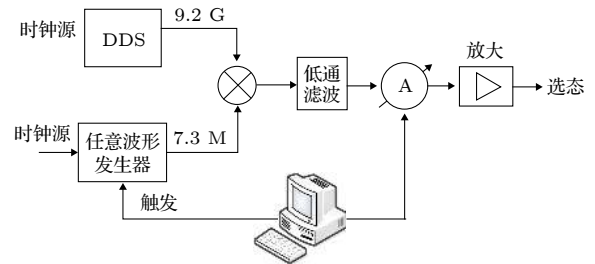
图 2 生成 RAP 脉冲的微波电路
