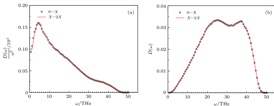
图 7 CuZr 金属玻璃 10 K 下通过对其原子的速度自关联函数进行傅里叶变换所得到的振动态密度, 数据表明 10 K 下系统内部已经几乎不存在可能影响到 D(\omega) 的老化过程
