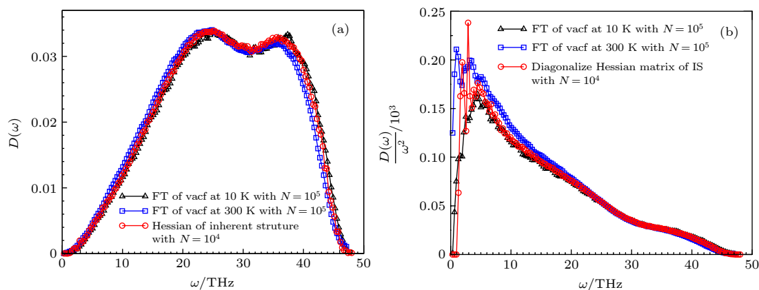
图 6 针对 CuZr 玻璃的不同粒子数及不同计算方法所获得的振动态密度 D(\omega) 的比较, 及对玻色峰的展示 [49]
