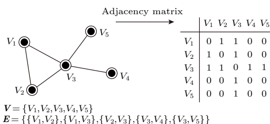
图 3 图或网络的示例以及它的邻接矩阵 [44]
