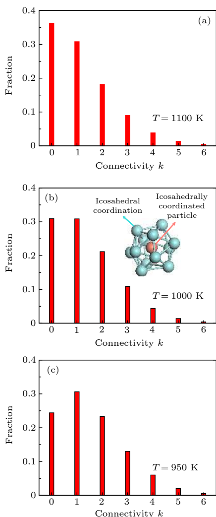
图 9 不同温度下二十面体中心原子的连接度的分布 [49]
