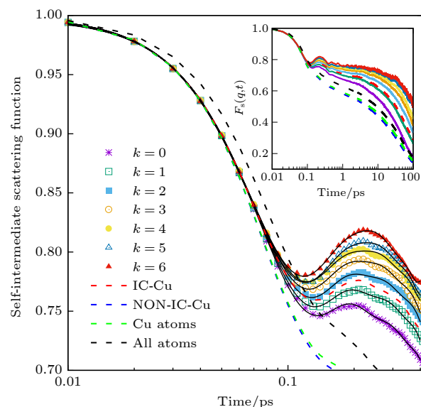
图 11 具有不同 k 值的粒子的自散射函数 (SISF) [49] , 图中黑色实线为唯象模型 ((9) 式) 的拟合结果, 图的右上角给出 SISF 曲线的整体形状; 其他类型粒子的 SISF 曲线也一并并在图中给出, 以方便对比
