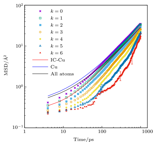
图 16 1000 K 下标记为不同类型的原子的均方位移曲线 [49]
