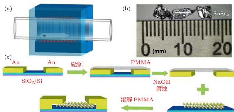
图 1 (a) 化学气相运输示意图; (b) \text{SnSe}_2 单晶; (c) 图形转移法流程图
