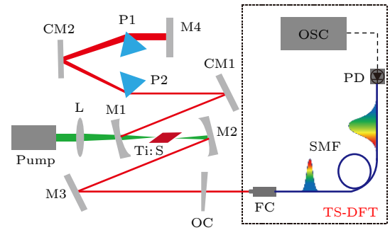
图 1 基于钛宝石激光器的 TS-DFT 实验装置图 (OC, 输出耦合镜; P, 棱镜对; CM, 啁啾镜对; L, 透镜; Ti:S, 钛蓝宝石晶体; M, 平面镜; FC, 光纤耦合器; SMF, 单模光纤; PD, 光电探测器; OSC, 高速示波器)
