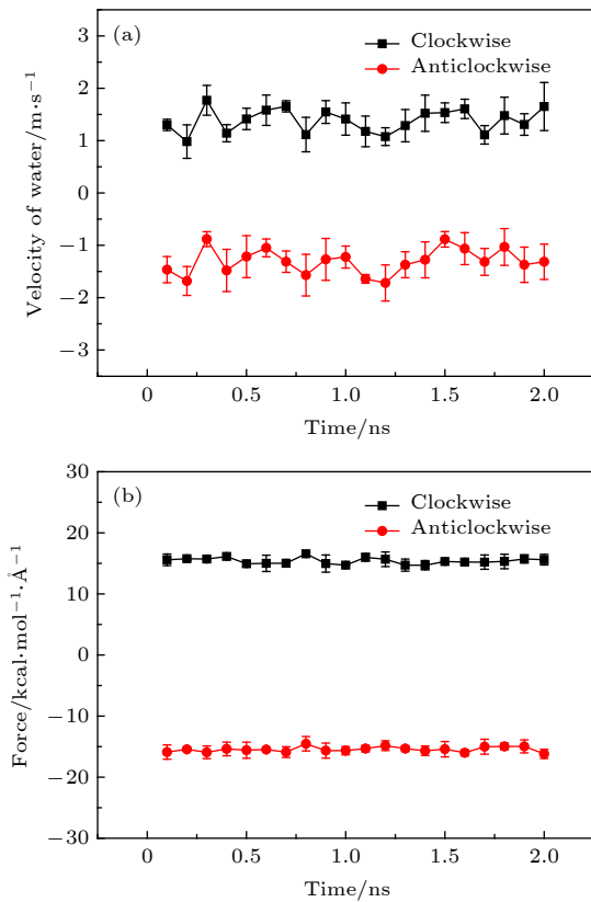
图3 手性角度为 23.4^\circ 的黑磷纳米管以 50 \text{ rad/ns} 的转速沿不同方向旋转时管内水分子沿轴向上的 (a) 速度和 (b) 受力随时间的变化关系
