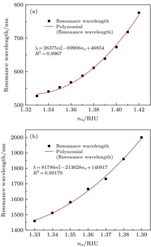
图 6 待测物 RI 与共振波长之间的关系 (a) 金膜厚度为 40 nm; (b) ITO 膜为 100 nm
