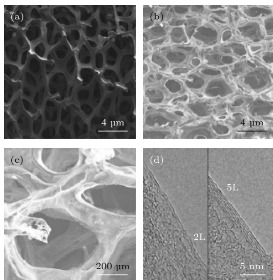
图 7 样品 SEM 图像 (a) 低压封闭 CVD 方法制备的 G/Ni 泡沫; (b) 低放大倍数的自支撑 3D GF; (c) 高放大倍数的自支撑 3D GF; (d) 石墨烯片边缘的高分辨 TEM 图像, 双层 (2 L) 和五层 (5 L) 石墨烯的层间距约为 0.33 nm, 样品由 500 \mu L PMMA 添加量制备
