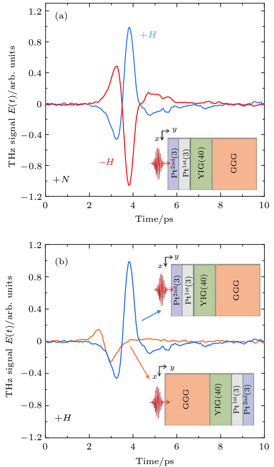
图 3 (a) 外加磁场 +H (蓝线) 和 -H (红线) 时, GGG//YIG(40)/Pt 1st (3)/Pt 2nd (3) 结构辐射的 THz 脉冲; (b) GGG//YIG(40)/Pt 1st (3)/Pt 2nd (3) 结构在不同激光激发装置下产生的 THz 脉冲,此时外加磁场固定为 +H , 插图: 飞秒脉冲激发样品的方向
