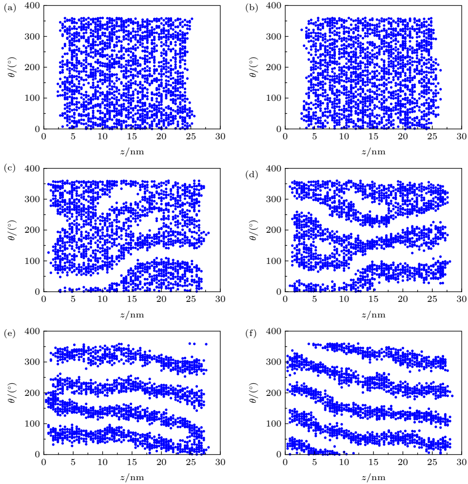
图 D1 d = 4 \text{ nm} 和 D = 4k_B T 时 GNRs 表面修饰剂的投影展开分布图, 其中摩尔比分别为 (a) 1:1, (b) 3:2, (c) 4:1, (d) 8:1, (e) 16:1, (f) 1:0
