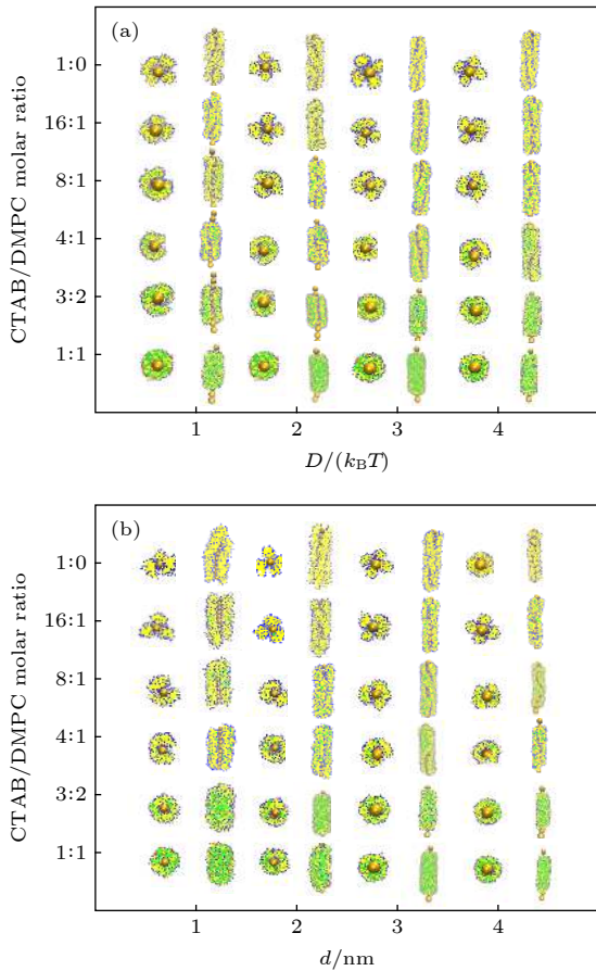
图 4 (a) 当金纳米棒直径 d = 4 \text{ nm} 时, GNRs-CTAB-DMPC 复合体在不同 CTAB/DMPC 摩尔比及 D 下的组装形貌; (b) 当 Morse 势参数 D = 4k_B T 时, GNRs-CTAB-DMPC 复合体在不同 CTAB/DMPC 摩尔比及 d 下的组装形貌
