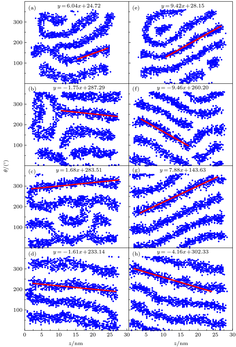
图 9 不同 D 下得到的 GNRs 表面修饰剂的投影展开分布图 (GNRs 直径 d = 4 nm), 其中, 线性拟合斜率代表螺旋程度; 左图是 CTAB/DMPC 摩尔比为 16:1 的结果, (a) D = 1k_B T , (b) D = 2k_B T , (c) D = 3k_B T , (d) D = 4k_B T ; 右图是 CTAB/DMPC 摩尔比为 1:0 的结果, (e) D = 1k_B T , (f) D = 2k_B T , (g) D = 3k_B T , (h) D = 4k_B T
