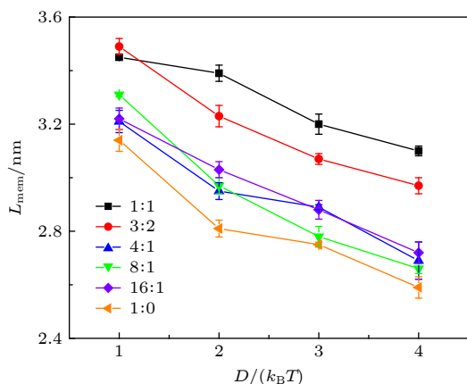
图 8 不同 CTAB/DMPC 摩尔比下得到的膜厚度 L_{mem} 与 D 的关系图.
