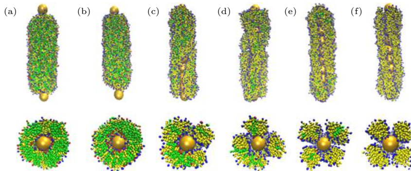
图 3 GNRs-CTAB-DMPC 复合体在 d = 4 nm, D = 4k_B T 时的组装形貌, 其中 CTAB/DMPC 摩尔比分别为 (a) 1:1, (b) 3:2, (c) 4:1, (d) 8:1, (e) 16:1, (f) 1:0
