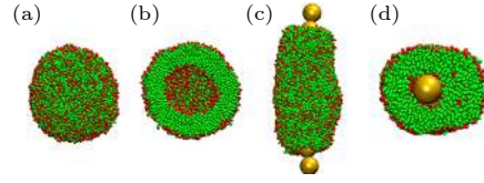
图 C1 纯 DMPC 和 d = 4 \text{ nm} , D = 4k_B T 时 GNRs-DMPC 的组装形貌 (a) DMPC 的形貌及 (b) 切面图; (c) GNRs-DMPC 的形貌及 (d) 切面图
