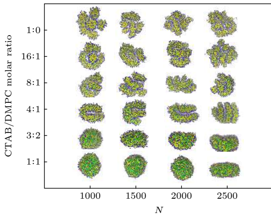
图 2 CTAB 和 DMPC 混合物的形貌图 (CTAB 的头部 H 和尾巴 T 珠子分别用蓝色和黄色表示, 而 DMPC 的 H 和 M/T 珠子分别用红色和绿色表示)
