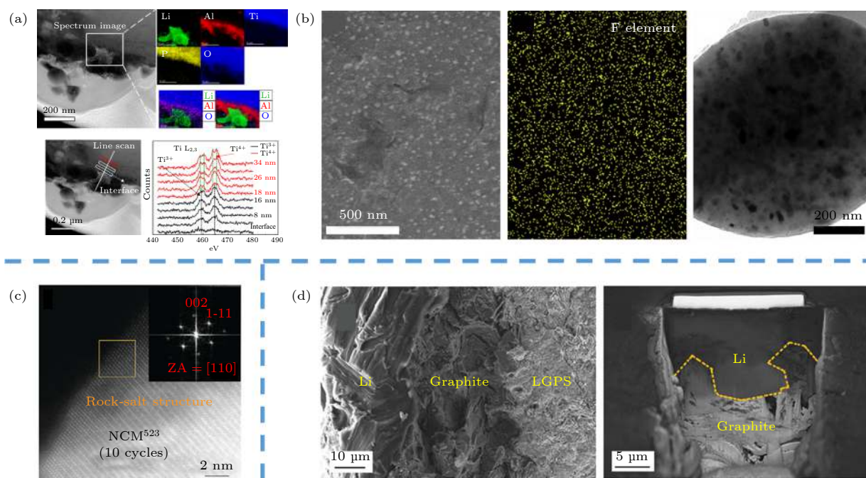
图5 电极和电解质的表面改性处理 (a) LAGP 固体电解质的表面包覆处理 [20] ; (b) LBH 固体电解质的原位 LiF 表面修饰 [21] ; (c) NCM523 正极的表面包覆处理 [22] ; (d) 金属锂负极的表面处理 [24] .
