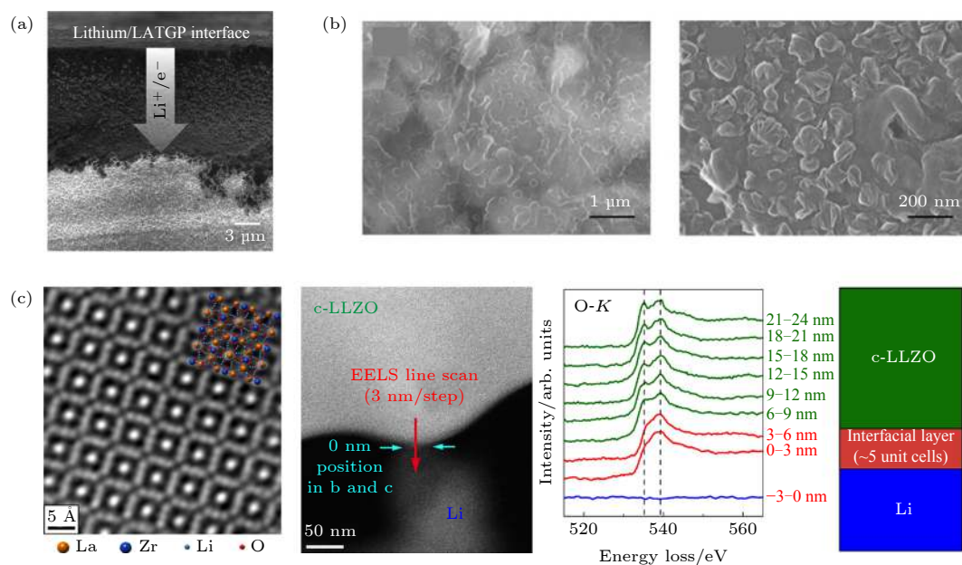
图 3 化学接触界面的结构和物质运输 (a) Li/LAGP 界面发生反应 [15] ; (b) Li/LZPO 界面反应 [16] ; (c) Li/LLZO 界面反应 [17]
