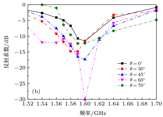
图 9 测量结果 (a) TE 波照射; (b) TM 波照射
