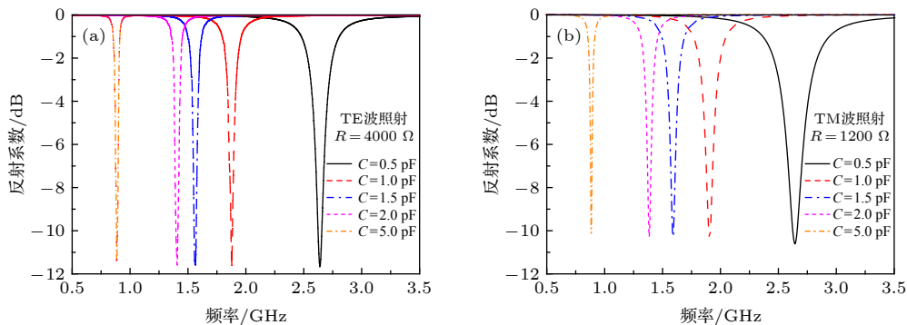
图 2 超材料吸波体的谐振频率随电容的变化 (a) TE 波照射; (b) TM 波照射
