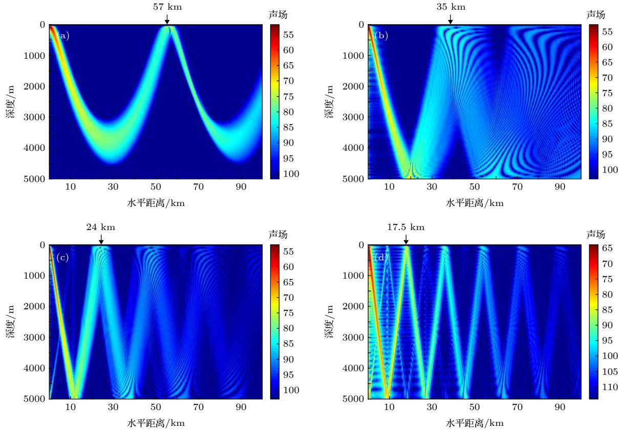
图 4 不同简正波 (声线) 簇形成的声场 (a) 1—120 阶简正波 (出射角 0^\circ — 9.5^\circ 的声线) 叠加声场; (b) 121—216 阶简正波 (出射角 9.5^\circ — 18.2^\circ 的声线) 叠加声场; (c) 217—314 阶简正波 (出射角 18.2^\circ — 27.6^\circ 的声线) 叠加声场; (d) 315—354 阶简正波 (出射角 27.6^\circ — 31.7^\circ 的声线) 叠加声场
