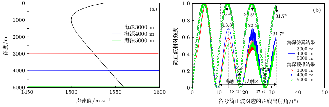
图 10 海深变化时声场角谱域分布 WKBZ 仿真结果和理论预报结果比较 (a) 不同海深下声速剖面; (b) 结果比较
