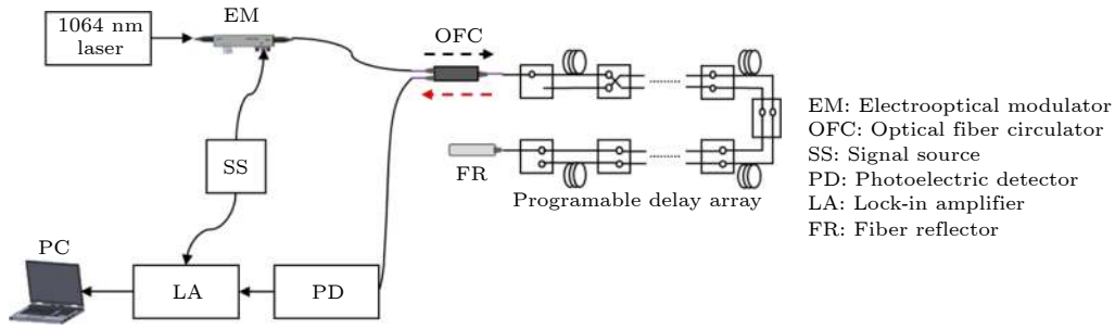
图 3 频域反射法测量光纤延时实验流程图
