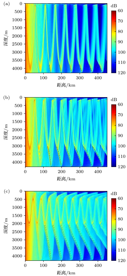
图 9 不同声源深度时 RR 型声线所形成的焦散线结构示意图, 实线为正角度出射声线所形成的焦散线, 虚线为负角度出射声线所形成的焦散线 (a) 声源深度 100 m; (b) 声源深度 200 m; (c) 声源深度 500 m
