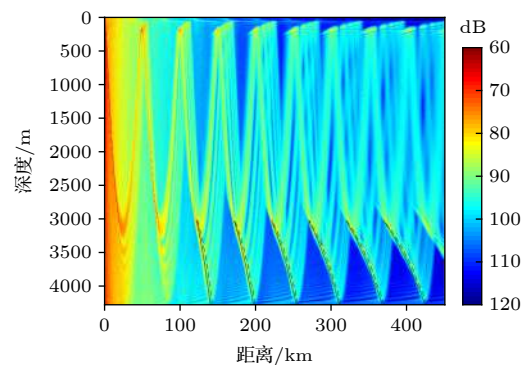
图 5 RR 型声线所形成的焦散线与传播损失伪彩图对比
