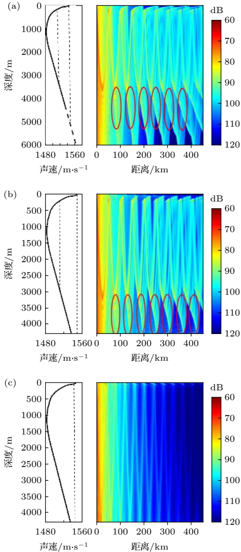
图 8 不同声速剖面传播损失对比图 (a) 完整声道; (b) 不完整声道声源深度声速小于海底声速; (c) 不完整声道声源深度声速大于海底声速
