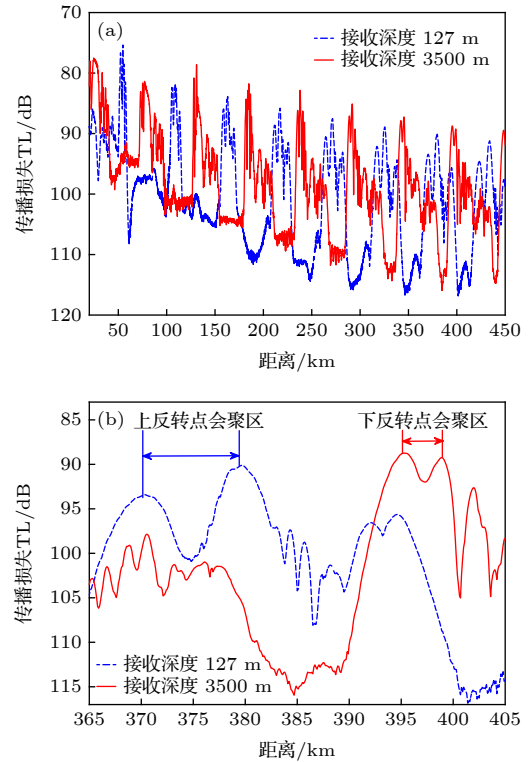
图 11 127 与 3500 m 接收深度传播损失对比 (a) 0—450 km; (b) 第 7 个会聚区处
