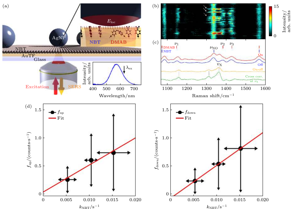
图 9 (a) “银纳米球-金膜”纳米腔体结构用于 SERS 测量及纳米腔暗场散射光谱 [65] ; (b) 催化反应生成中间产物的间歇性光谱特征轨迹 [65] ; (c) 在开 (红) 和关 (蓝) 期间从图 9(b) 中取样的 SERS 光谱, 两者光谱的差异 (橙) 及其协方差矩阵 V_X = 1364 \text{ cm}^{-1} 分量 (绿). 在 1160, 1314, 1364 \text{ cm}^{-1} 处出现间歇性 SERS 峰归因于中间产物羟胺基苯硫醇分子的拉曼峰 [65] ; (d) 光谱的上升沿阶跃频率 f_{\text{up}} (左) 和下降沿阶跃频率 f_{\text{down}} (右) 与 4-NTP 分子的衰减速率常数 k_{\text{NBT}} 之间的关系 [65]
