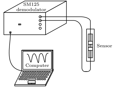
图 6 实验装置
