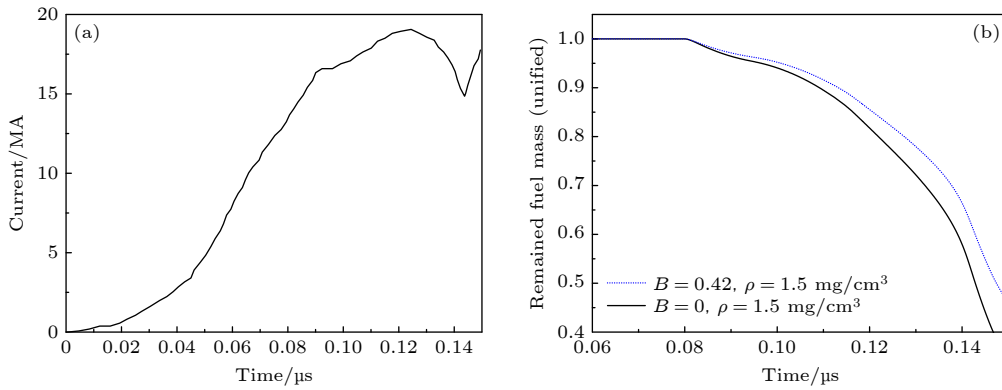
图 7 MIST 计算所使用的 (a) 驱动电流曲线, 以及 (b) 剩余燃料质量随时间演化曲线 Fig. 7. Demonstrations of (a) driving current and (b) remained fuel mass calculated by MIST.
