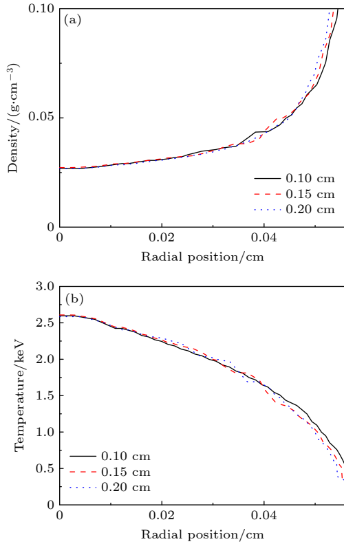
图 10 不同 LEH 半径下, MIST 计算得到的 139 ns 时的 (a) 密度分布和 (b) 温度分布 Fig. 10. Distributions of (a) density and (b) temperature calculated by MIST under different LEH radii at 139 ns.
