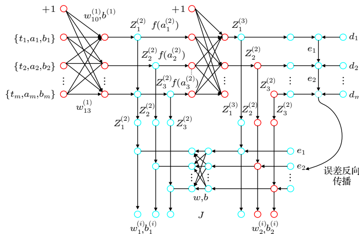
图 5 BP 神经网络时钟同步误差补偿结构图
