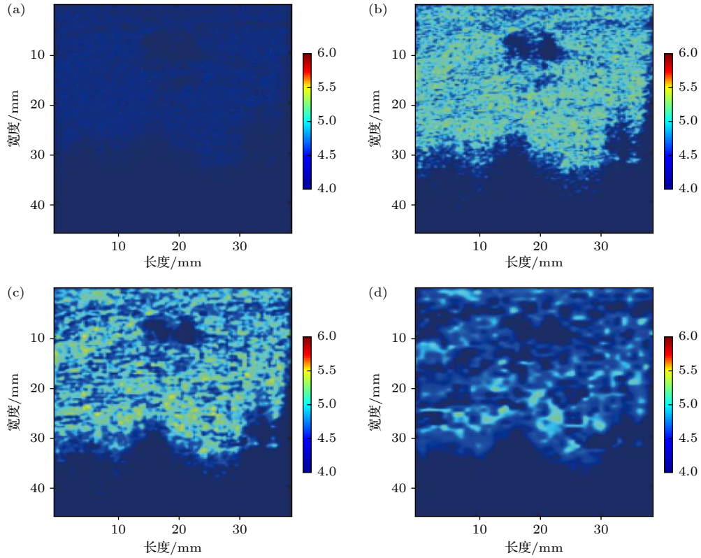
图 6 不同滑动窗口大小重构的熵图 (a) 0.2 倍脉冲长度; (b) 0.5 倍脉冲长度; (c) 1.0 倍脉冲长度; (d) 2.0 倍脉冲长度
