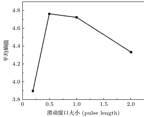
图 7 306 例乳腺 RF 信号的平均熵值随窗口大小的变化 Fig. 7. Dependence of averaged entropy on window size for 306 samples.
