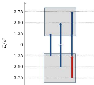
图2 多光子跃迁过程示意图, 外场频率为 \omega = 2.5c^2
