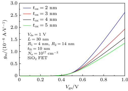
图 12 不同 SiO 2 栅介质厚度下的跨导
