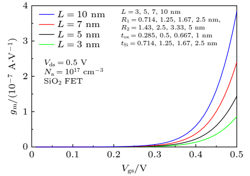
图 15 不同栅长下的跨导
