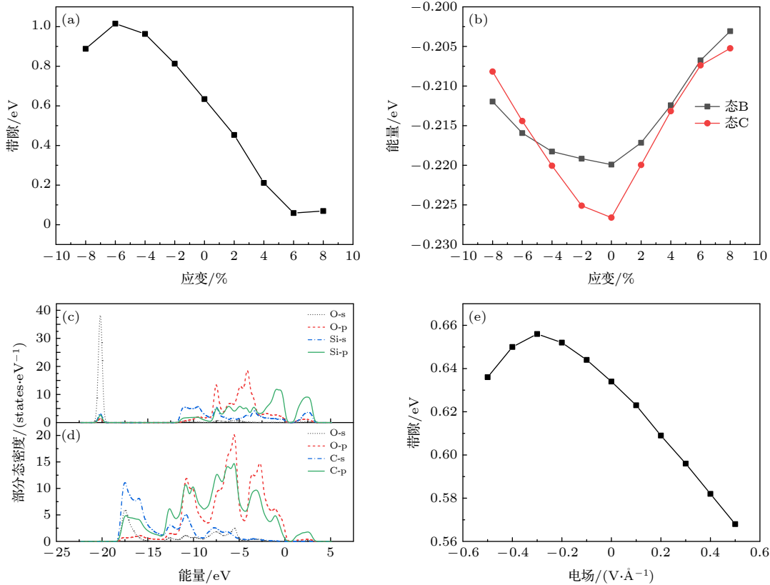
图 5 (a) 双轴应变下硅醚/石墨醚异质结构的带隙变化; (b) 双轴应变下态 B 和态 C 的能量; 应变为 -6% 时异质结构中 (c) 硅醚和 (d) 石墨醚的 PDOS 图; (e) 不同垂直电场强度下带隙变化
