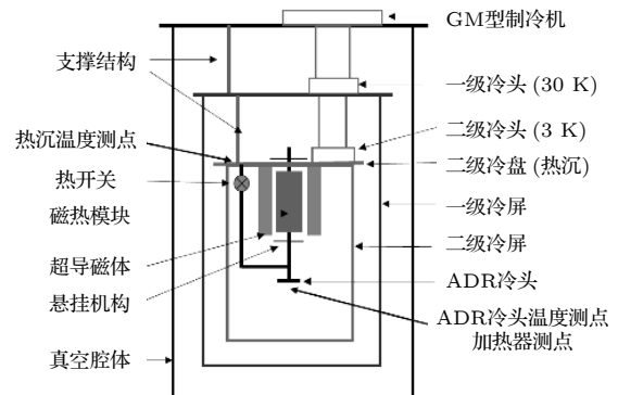
图 3 制冷系统示意图 Fig. 3. Schematic diagram of refrigeration system.
