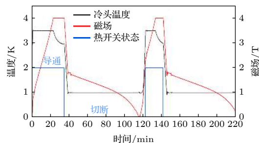
图 6 典型的 ADR 工作过程
