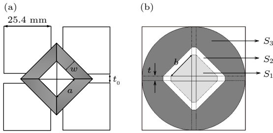
图 1 加载前后八面腔压机密封边的形态示意图 (a) 加载前的预密封条; (b) 加载后预密封条受挤压流动形成的密封边区域
