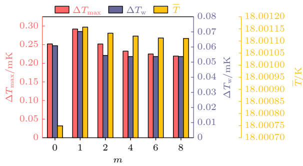
图 9 不同光纤数量下靶丸外表面最大温差、加权温差及平均温度变化 Fig. 9. \Delta T_{max} , \Delta T_w and \bar{T} variations of capsule outside surface responding to optical fiber numbers.
