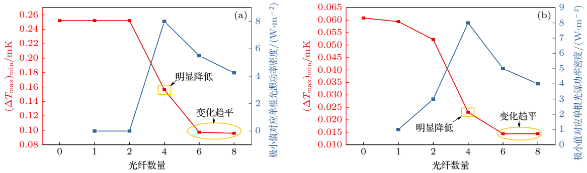
图 13 不同光纤数量下, 靶丸外表面最大温差极小值和加权温差的极小值及其对应的光源功率密度的变化曲线 (a) 最大温差极小值; (b) 加权温差的极小值
