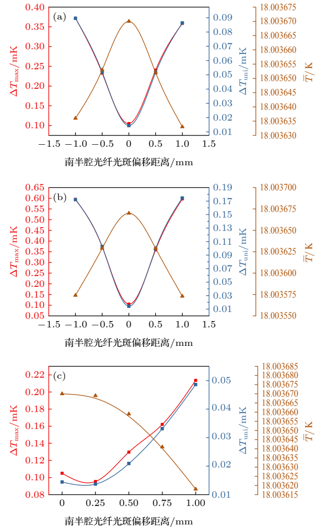
图 16 3 种方案下靶丸外表面最大温差、加权温差和平均温度随南半腔光纤光斑偏移距离变化曲线 (a) 方式 1; (b) 方式 2; (c) 方式 3 Fig. 16. \Delta T_{\max} , \Delta T_w and \bar{T} variations with migration distance of southern half hohlraum IR spots corresponding to 3 kinds of IR spots offsets: (a) Model1; (b) mode2; (c) mode3.
