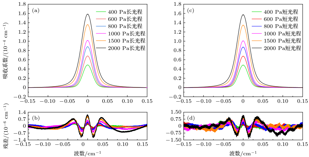
图 7 (a), (b) 在长光程中 9152.53 \text{ cm}^{-1} 处纯水分子的吸收系数和拟合残差; (c), (d) 在短光程中纯水分子在相同光谱线位置的吸收系数和拟合残差
