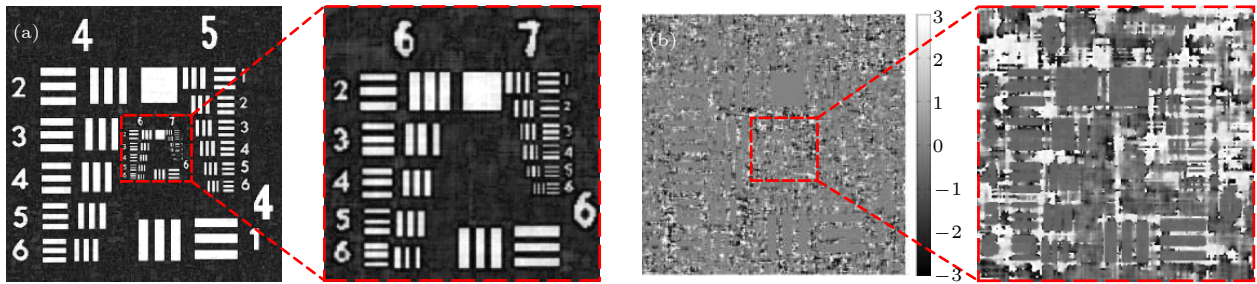
图 4 同轴全息图再现结果 (a) 振幅像; (b) 相位像 Fig. 4. Reconstructed results of in-line hologram: (a) Amplitude image; (b) phase image.
