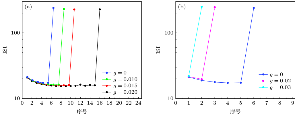
图 4 不同自突触电导下的簇放电的峰峰间期 ISI 随序号的变化 (a) 抑制性自突触, g = 0 (蓝), g = 0.01 (绿), g = 0.015 (红) 和 g = 0.02 (黑); (b) 兴奋性自突触, g = 0 (蓝), g = 0.02 (粉) 和 g = 0.03 (青)
