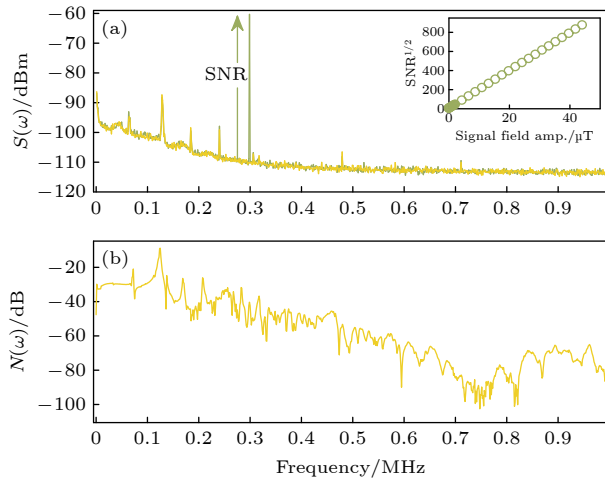
图 7 (a) 电光调制频率为 15 MHz 时的功率谱密度 S(\omega) ; 绿色峰为 280 kHz 处的参考磁场信号; 插图: \text{BW} = 330 Hz 时 SNR 开方值随信号场强度变化关系; (b) 系统响应 N(\omega)
