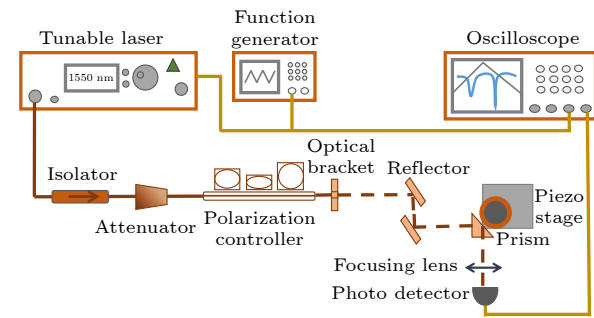
图 4 光学品质因数测量实验装置图
