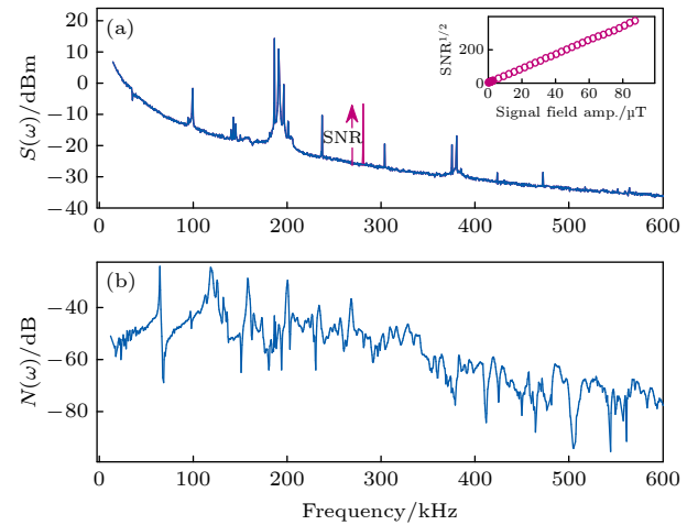
图 8 (a) 电光调制频率为 13.6 MHz 时的功率谱密度 S(\omega) , 280 kHz 参考磁场频率处有峰值响应; 插图: \text{BW} = 10 Hz 条件下, SNR 开方值随信号场强度变化关系; (b) 系统响应 N(\omega)
