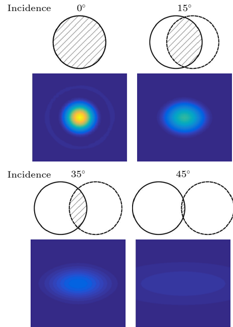
图 9 镀膜角锥棱镜不同入射角的 FFDP (图样范围约 16'' \times 16'' )
