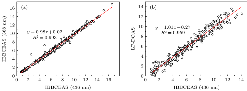
图 6 (a) IBBCEAS (中心波长 368 nm) 和 IBBCEAS (中心波长 436 nm) 测量的 NO 2 浓度的相关性; (b) IBBCEAS (中心波长 436 nm) 和 LP-DOAS 测量的 NO 2 浓度的相关性
