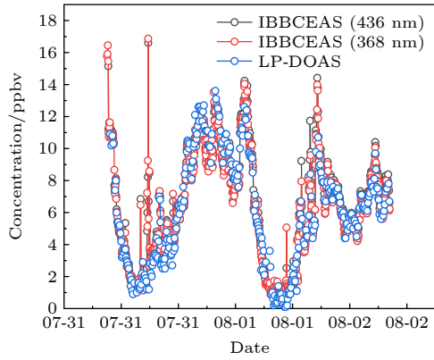
图 5 三套系统测量的 NO 2 浓度时间序列图, 黑线为中心波长为 436 nm 的 IBBCEAS 系统的 NO 2 浓度时间序列, 红线为中心波长为 368 nm 的 IBBCEAS 系统的 NO 2 浓度时间序列, 蓝线为 LP-DOAS 系统的 NO 2 浓度时间序列
