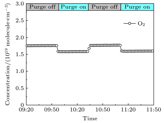
图 3 依次关闭和开启 N_2 吹扫时测量的 O_2 浓度时间序列图
