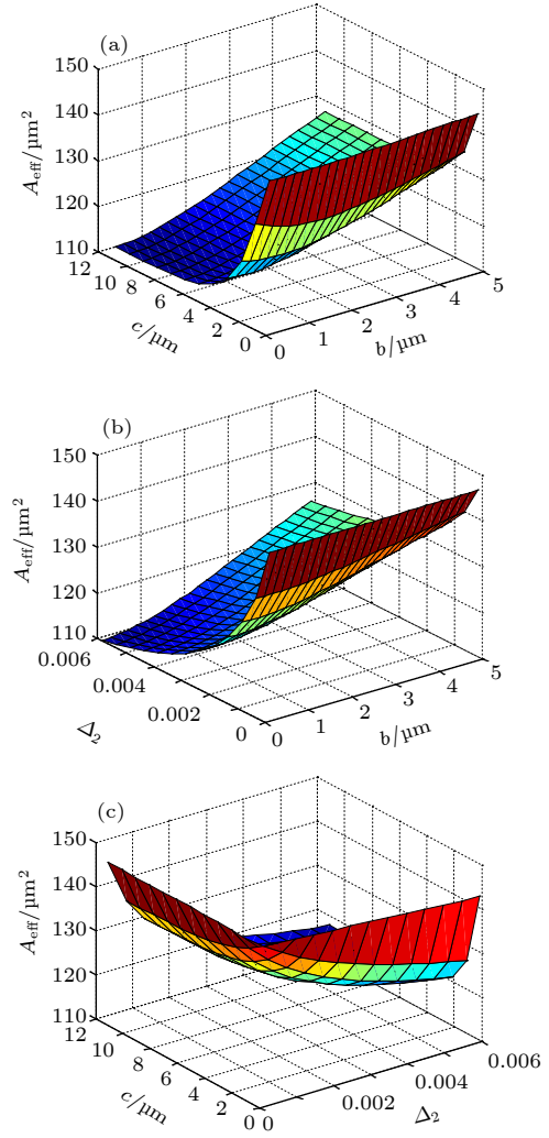
图 6 A_{\text{eff}} 随不同层结构参数 (a) b 和 c 、(b) b 和 \Delta_2 和 (c) \Delta_2 和 c 的变化关系
