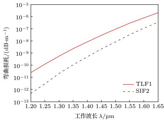
图 10 TLF 基模的限制损耗随波长的变化曲线 Fig. 10. Transmission loss of fundamental mode for TLFs.
