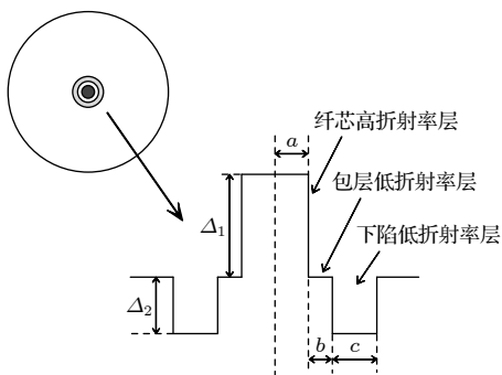
图 1 TLF 的横截面结构及折射率分布图
