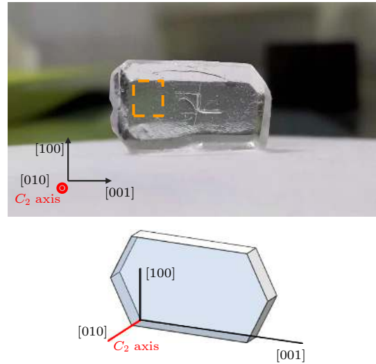
图 1 \text{EuCl}_3 \cdot 6\text{H}_2\text{O} 晶体, 厚度约 2 mm, 虚线内为存储实验所用区域. 晶体的三个轴向标示在示意图中, C_2 轴沿晶体的 [010] 的方向
