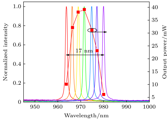
图 9 用 6 mm 厚度 BRF 作调谐元件的 SDL 的调谐特性 Fig. 9. Tuning characteristics of the SDL with 6 mm thickness BRF.
