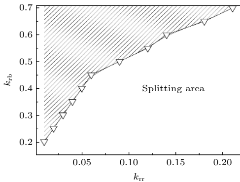
图 2 反射谱无分裂峰时 k_{rb} 和 k_{rr} 的关系
