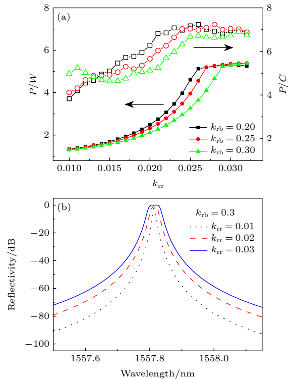
图 7 (a) 耦合系数与 P/W , P/C 的关系; (b) k_{rb} = 0.3 时, 不同 k_{rr} 取值下, 反射谱特性
