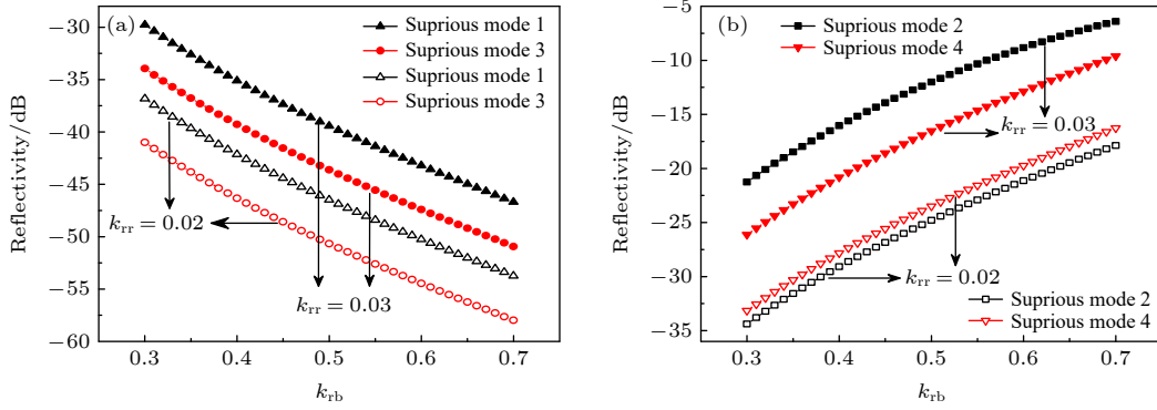
图 4 哑铃型微腔伪模的峰值透射率变化与 k_{rb} 的关系 (a) 伪模 1 和 3 随耦合系数的变化曲线; (b) 伪模 2 和 4 随耦合系数的变化曲线 Fig. 4. Peak reflection of different spurious modes versus k_{rb} : (a) Reflectivity of spurious mode 1 and 3 versus k_{rr} and k_{rb} , respectively; (b) reflectivity of spurious mode 2 and 4 versus k_{rr} and k_{rb} , respectively.
