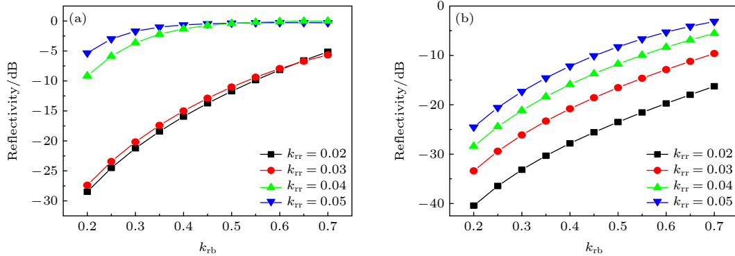
图 5 耦合系数 k_{rb} 与伪模 2, 4 反射率的关系 (a) 伪模 2; (b) 伪模 4
