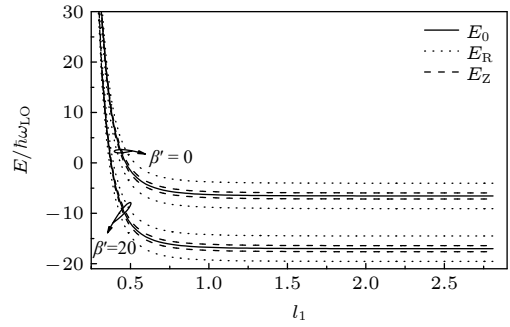
图 1 取固定值 \omega_c = 1\omega_{LO} , l_2 = 1.2 , \alpha = 8 , \alpha_R = 1 , 当库仑束缚势 \beta' 取不同值时, 束缚磁极化子基态能量 E 与横向有效受限长度 l_1 之间的关系曲线
