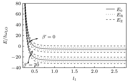
图 3 取固定值 \omega_c = 10\omega_{LO} , l_2 = 1.2 , \alpha = 8 , \alpha_R = 1 , 当库仑束缚势 \beta' 取不同值时, 束缚磁极化子基态能量 E 与横向有效受限长度 l_1 之间的关系曲线
