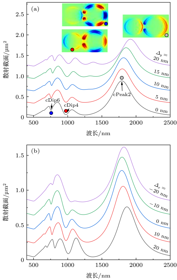
图 6 当 \varphi = 90^\circ 时二聚体的散射谱随 \Delta_x , \Delta_y 的变化 (a) \Delta_x = 0 nm, \Delta_y 从 0 nm 到 20 nm; (b) \Delta_y = 0 nm, \Delta_x 从 -20 nm 到 20 nm. 插图为 \Delta_x = 0 nm, \Delta_y = 20 nm 时的散射谱中指定频率处的二聚体表面电场分布
