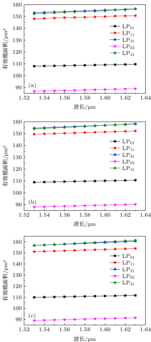
图 7 各 LP 模式在 C+L 波段的有效模面积变化情况 (a) 纤芯 1; (b) 纤芯 2; (c) 纤芯 3 Fig. 7. Effective mode area changes of each LP mode in the C+L band: (a) Core 1; (b) Core 2; (c) Core 3.
