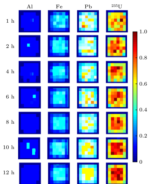
图 10 不同成像时间内物块模型成像结果
