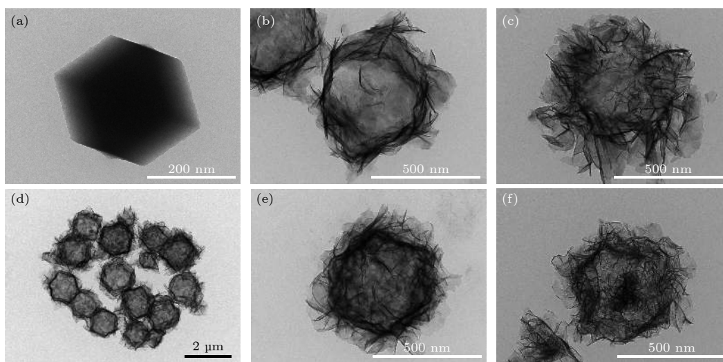
图 5 样品的透射电镜图 (a) ZIF-67; (b) Ni 0 Co 1 -LDH; (c) Ni 1 Co 1 -LDH; (d) Ni 2 Co 1 -LDH; (e) Ni 2 Co 1 -LDH; (f) Ni 1 Co 0 -LDH
