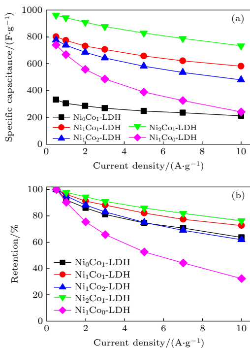
图 9 样品在不同电流密度下的 (a) 比电容和 (b) 电容保留率 Fig. 9. (a) Specific capacitances and (b) capacitance retentions of the samples under various current densities.
