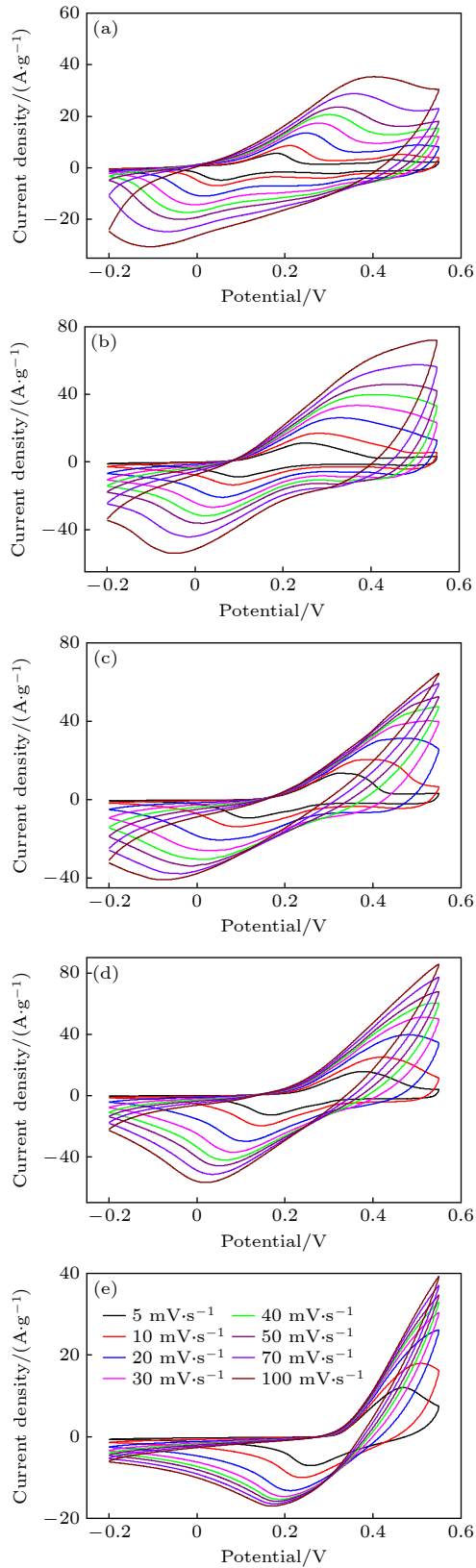
图7 样品在不同扫描速度下的循环伏安曲线 (a) \text{Ni}_0\text{Co}_1\text{-LDH} ; (b) \text{Ni}_1\text{Co}_2\text{-LDH} ; (c) \text{Ni}_1\text{Co}_1\text{-LDH} ; (d) \text{Ni}_2\text{Co}_1\text{-LDH} ; (e) \text{Ni}_1\text{Co}_0\text{-LDH}
