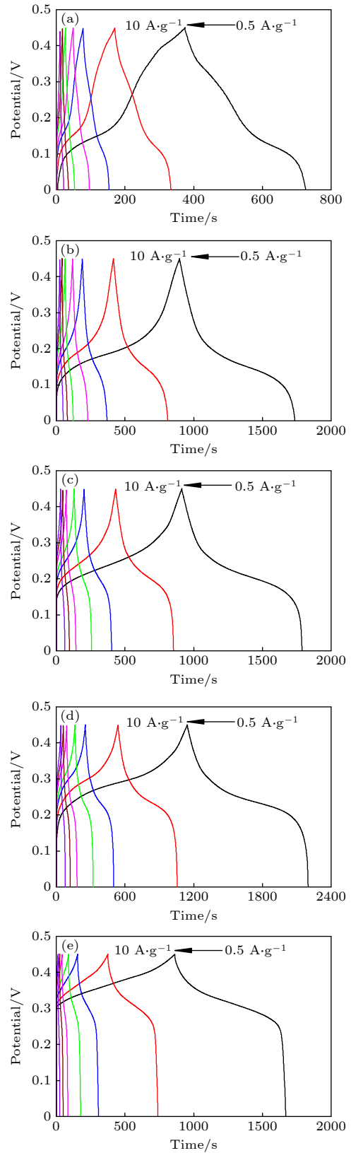
图8 样品在不同电流密度下的恒电流充放电曲线 (a) \text{Ni}_0\text{Co}_1\text{-LDH} ; (b) \text{Ni}_1\text{Co}_2\text{-LDH} ; (c) \text{Ni}_1\text{Co}_1\text{-LDH} ; (d) \text{Ni}_2\text{Co}_1\text{-LDH} ; (e) \text{Ni}_1\text{Co}_0\text{-LDH}
