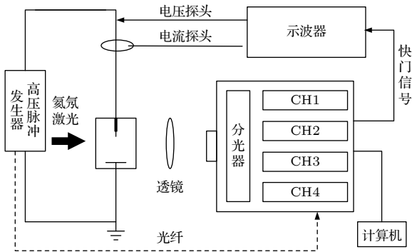
图 1 实验装置示意图 Fig. 1. Experimental setup.
