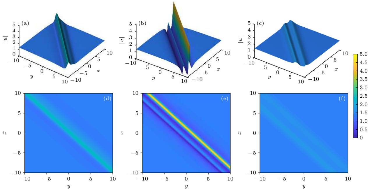
图 6 (a), (b), (c) 传播距离 z = -1, 0.29, 1.5 时二线怪波簇 |u| 在 x - y 平面上的三维图; (d), (e), (f) 对应的投影图; (a), (d) A = 2.76 ; (b), (e) A = 4.53 ; (c), (f) A = 1.72 ; 参数 w_0 = \gamma = \beta_0 = 1, \varsigma_0 = \zeta_0 = \varphi_0 = 0, \mu = 20, \delta = -20
