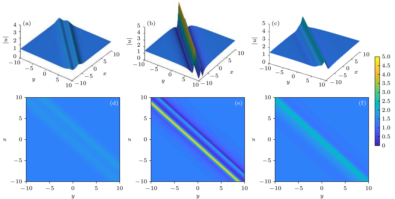
图 7 传播距离 z = -1.5, -0.295, 1 时二阶线怪波簇 |u| (a), (b), (c) 三维图; (d), (e), (f) 对应 x - y 面上的投影图; (a), (d) A = 1.72 ; (b), (e) A = 4.39 ; (c), (f) A = 2.39 ; 参数 w_0 = \gamma = \beta_0 = 1, \varsigma_0 = \zeta_0 = \phi_0 = 0, \mu = -20, \delta = 20
