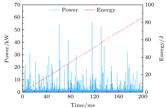
图10 常压下滑动弧放电的瞬时功率和能量
