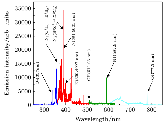
图 12 大气压滑动弧放电发射光谱
